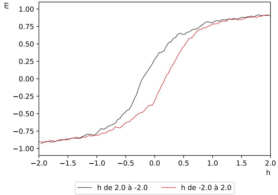
Hystérésis de l'aimantation - réseau de taille L=64 - champ magnétique d'amplitude h=2 à T=3.5
